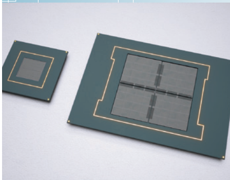
ICパッケージ基板
